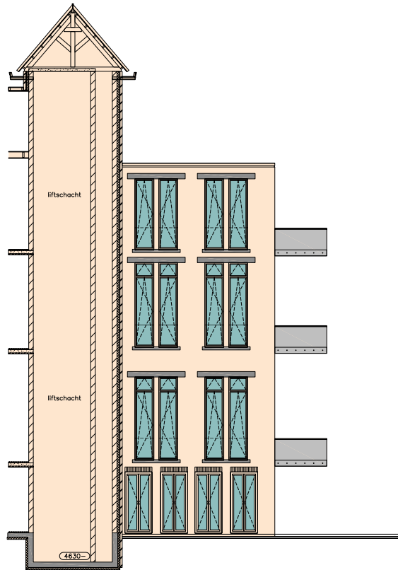
gevel H
