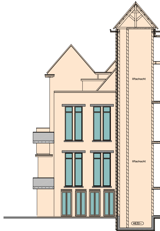
gevel J
